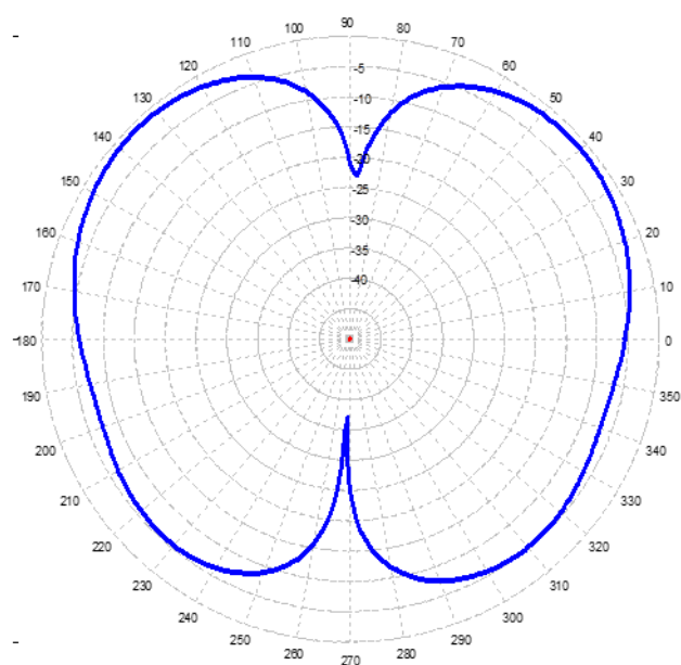
460 MHz
