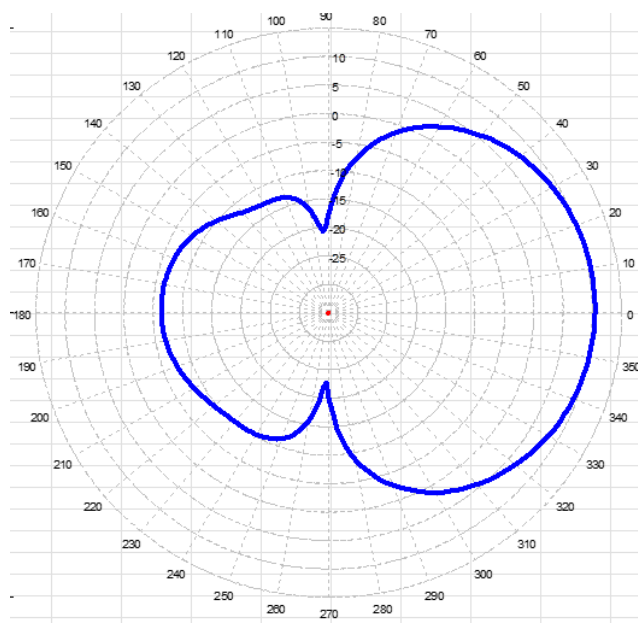
390 MHz
