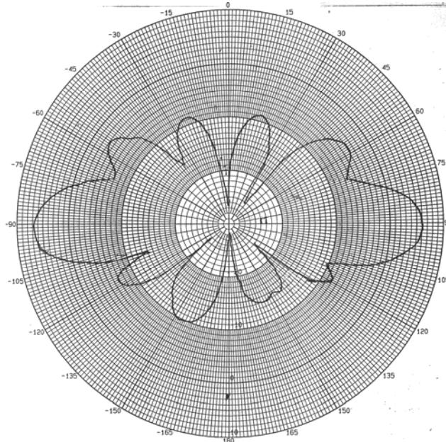
OD @ 1800 MHz– Elevation Plot
