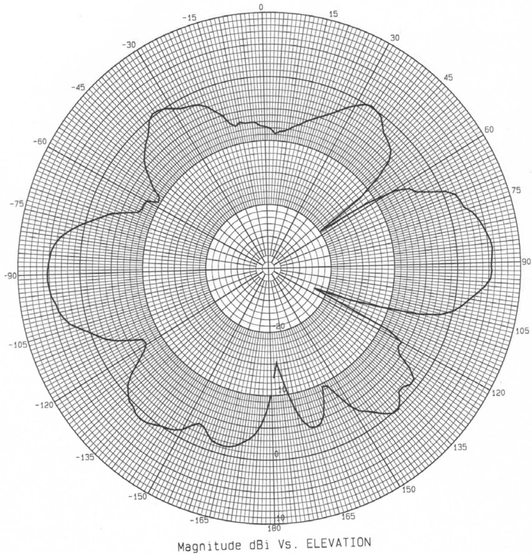
OD5-5900MOD2- Elevation
